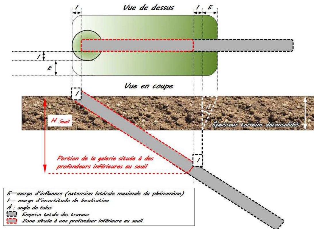
Illustration 12 : zonage de l'aléa effondrement localisé lié à la présence d'une galerie ou d'une descenderie souterraine (vue en plan)
