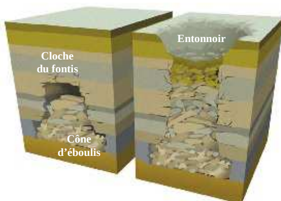
Illustration 4 : description du phénomène d'effondrement localisé
