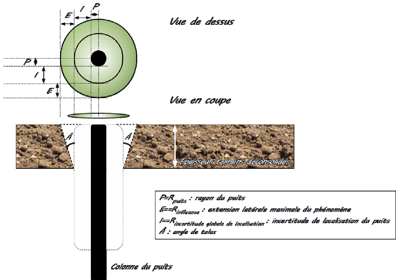
Illustration 11: zonage de l'aléa effondrement localisé lié aux puits
